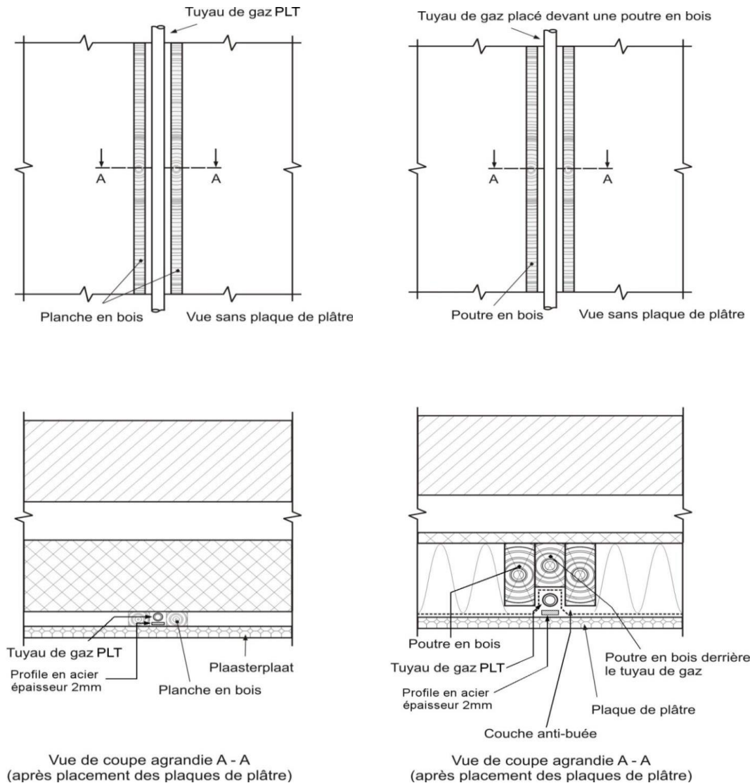
Configuration spatiale 4 : Exemple de tuyau de gaz derrière une paroi en plaques de plâtre
