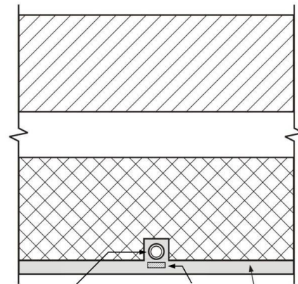
Tuyau de gaz PLT dans une découpe se trouvant dans un mur plâtré Profilé en acier épaisseur 2mm Plâtre
